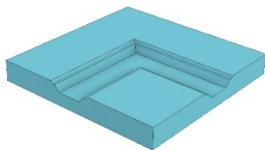
DESIGN : D16 GROOVE DEPTH : 5mm
